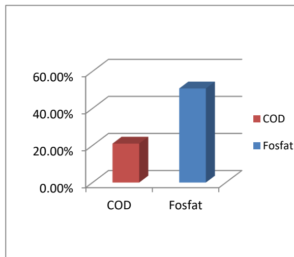
Gambar 1. Persentase Removal COD, dan Fosfat
